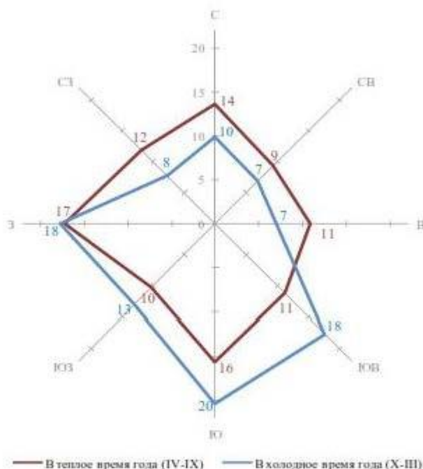
Рисунок 2. Повторяемость направлений ветра по периодам года, %
