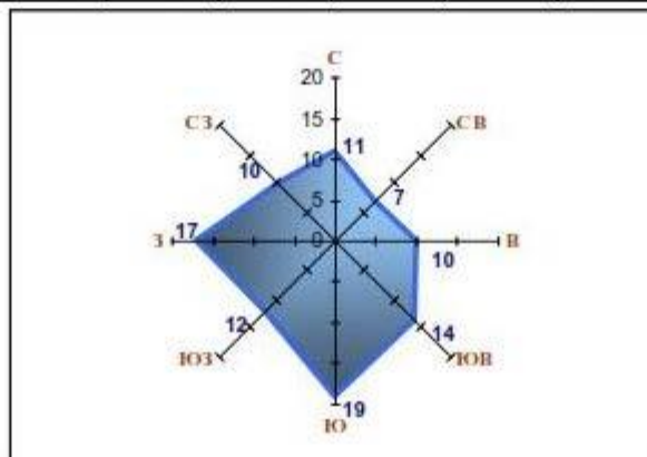
Рис. 1.6.1. Роза ветров территории
