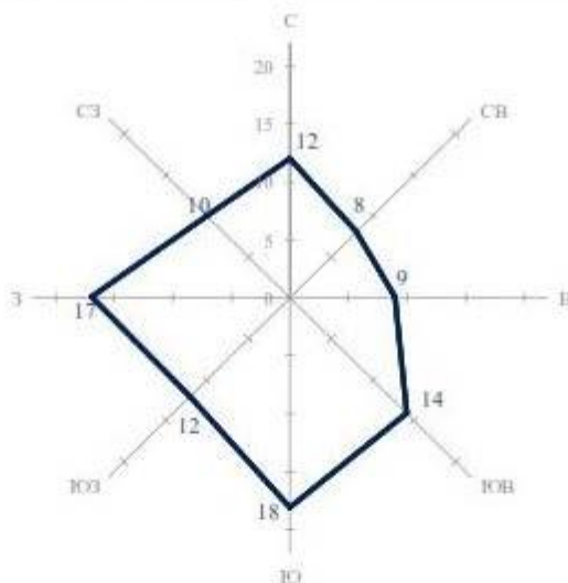
Рисунок 1. Роза ветров территории
